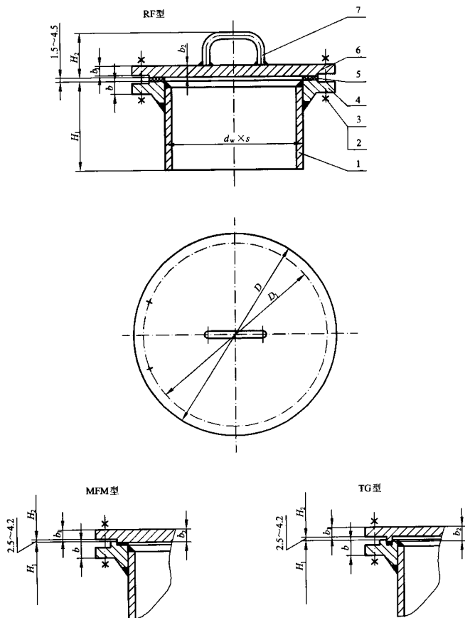
图 3 手孔的型式
