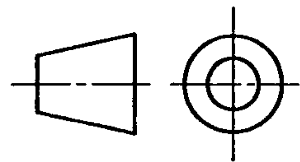
图 11 第一角画法的投影识别符号
