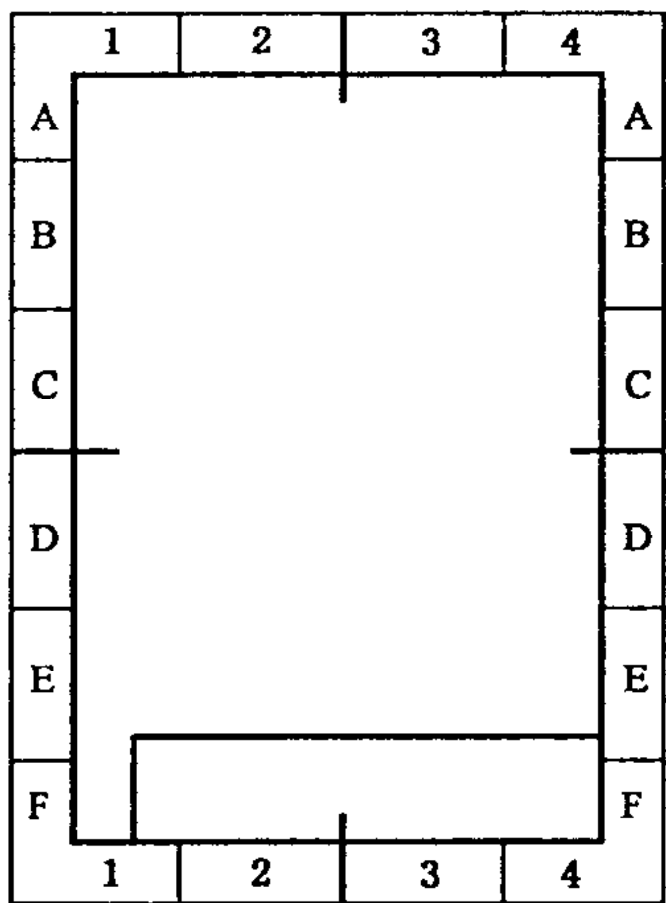
图 14 图幅分区(二)
