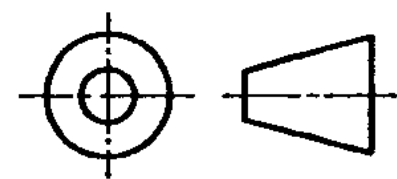
图 12 第三角画法的投影识别符号
