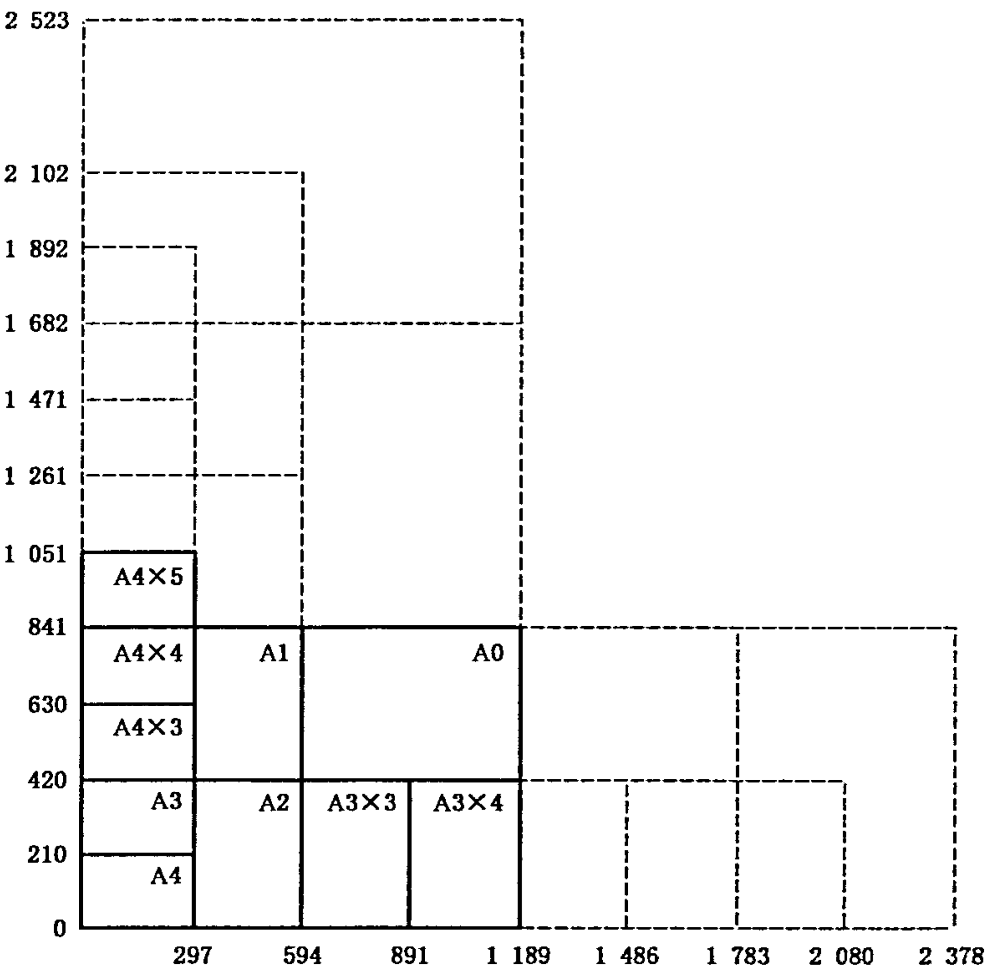
图 1 图纸的幅面尺寸
