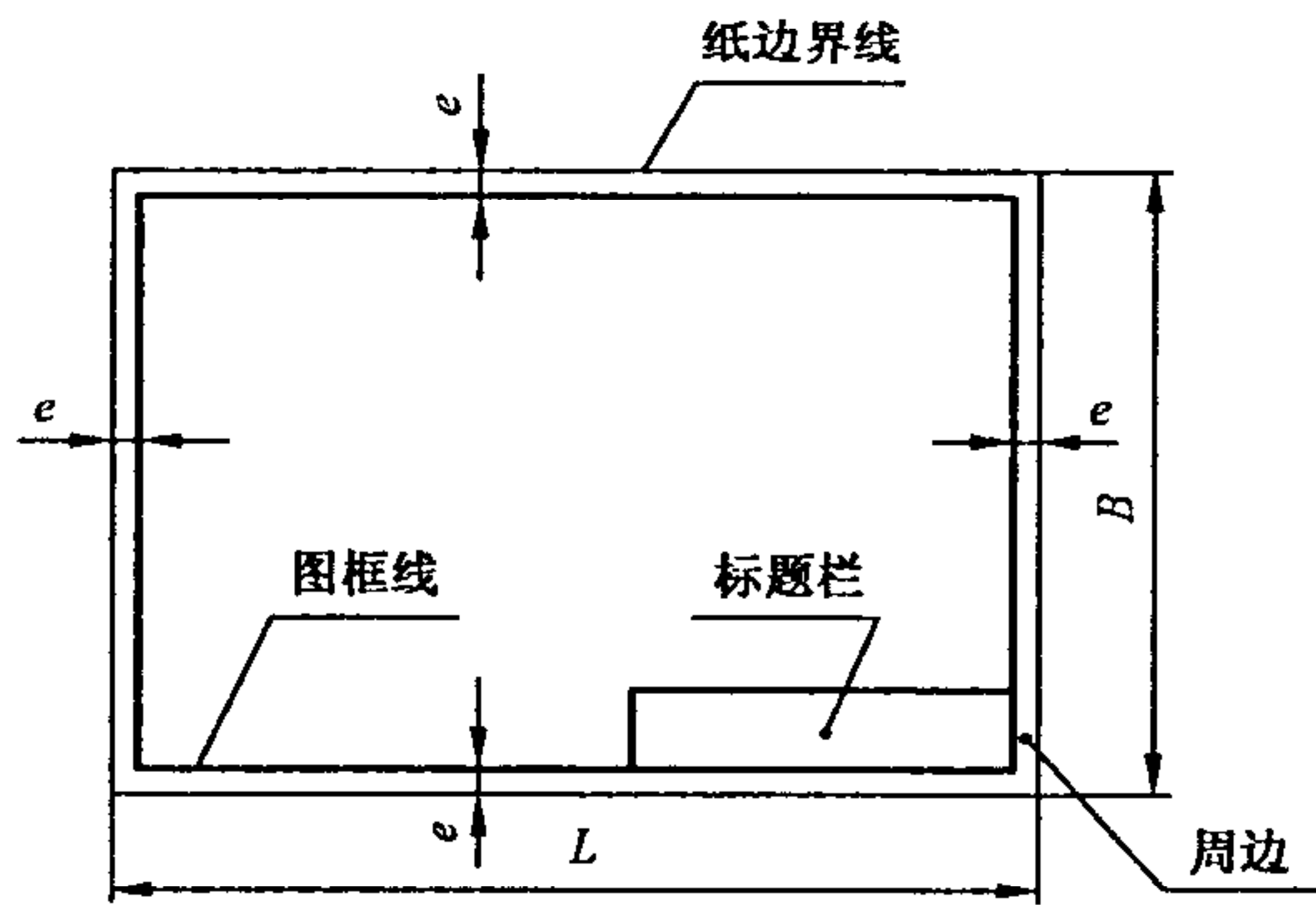
图 2 无装订边图纸(X 型)的图框格式
