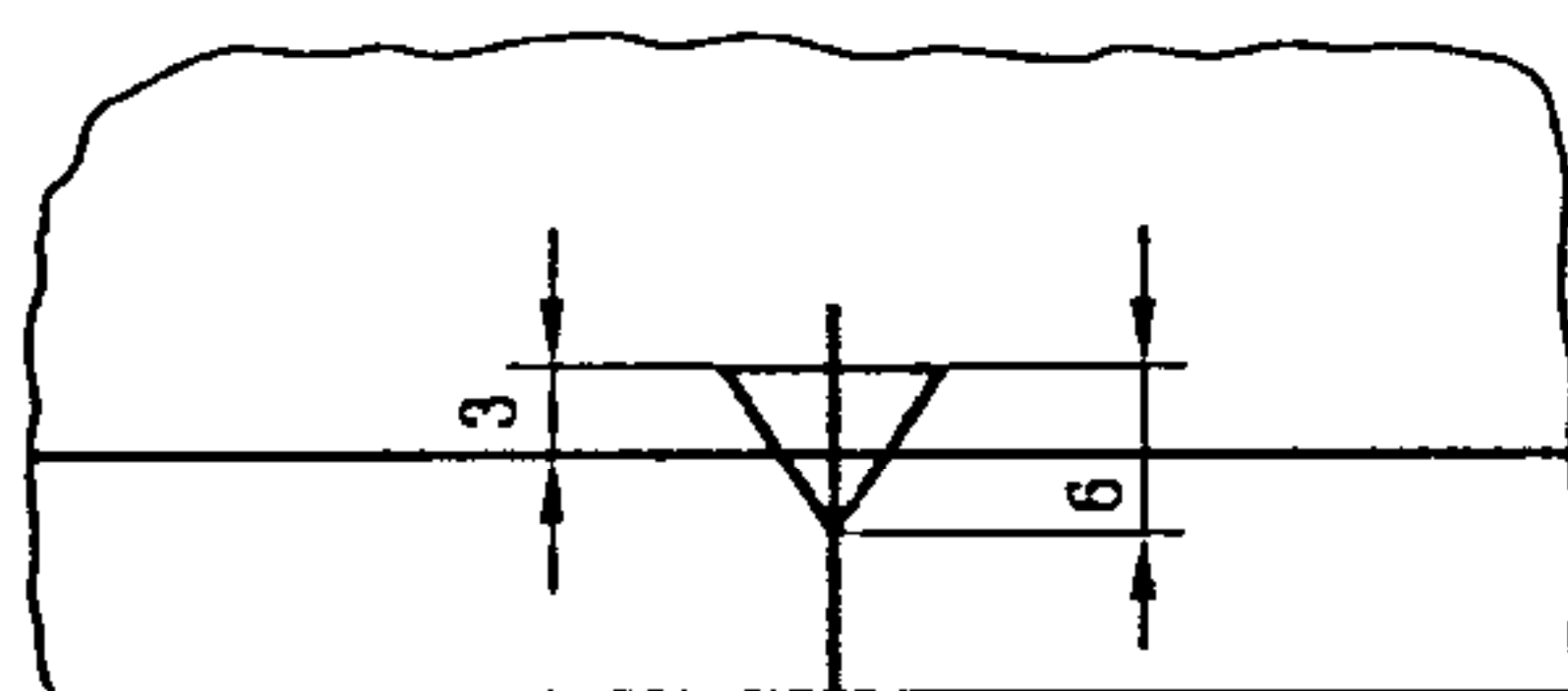
图8 方向符号的尺寸和位置
