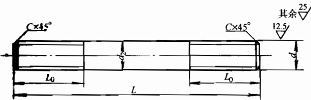
图1 A型螺柱
