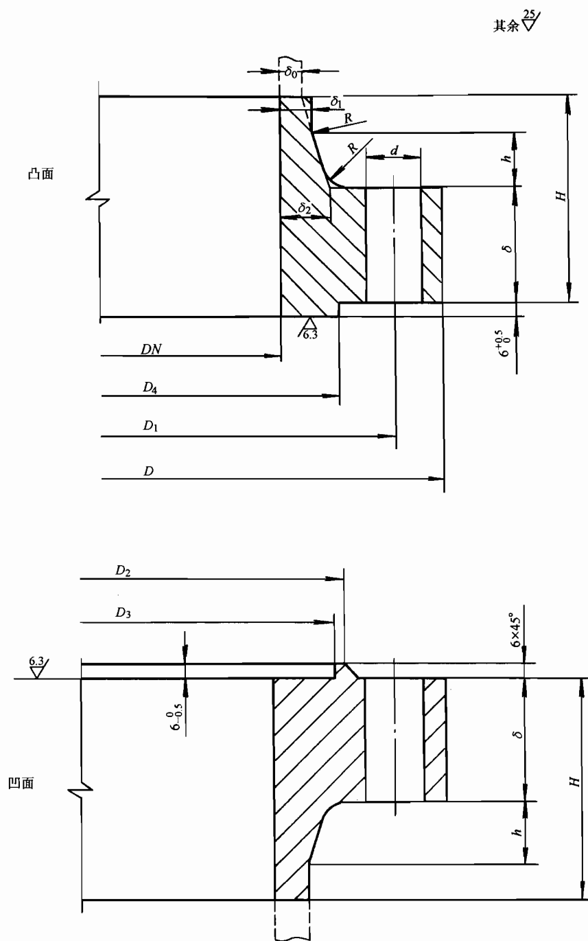
图 2 凹凸密封面
