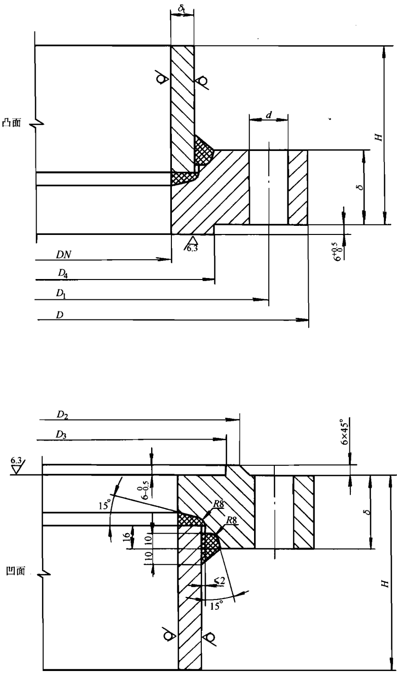
图 2 凹凸密封面
