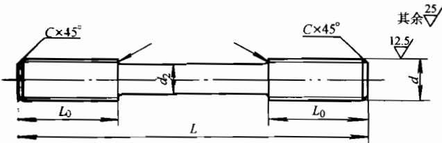
图2 B型螺柱
