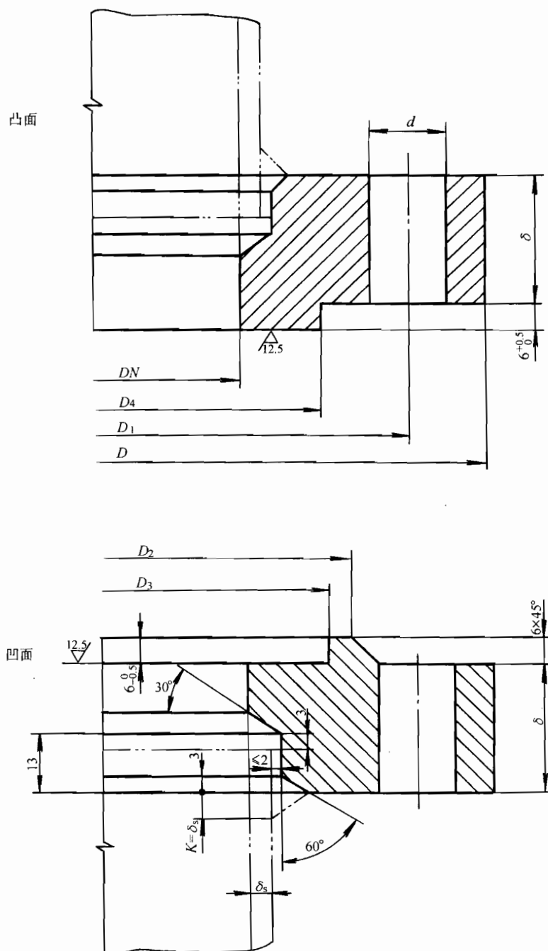
图 2 凹凸密封面
