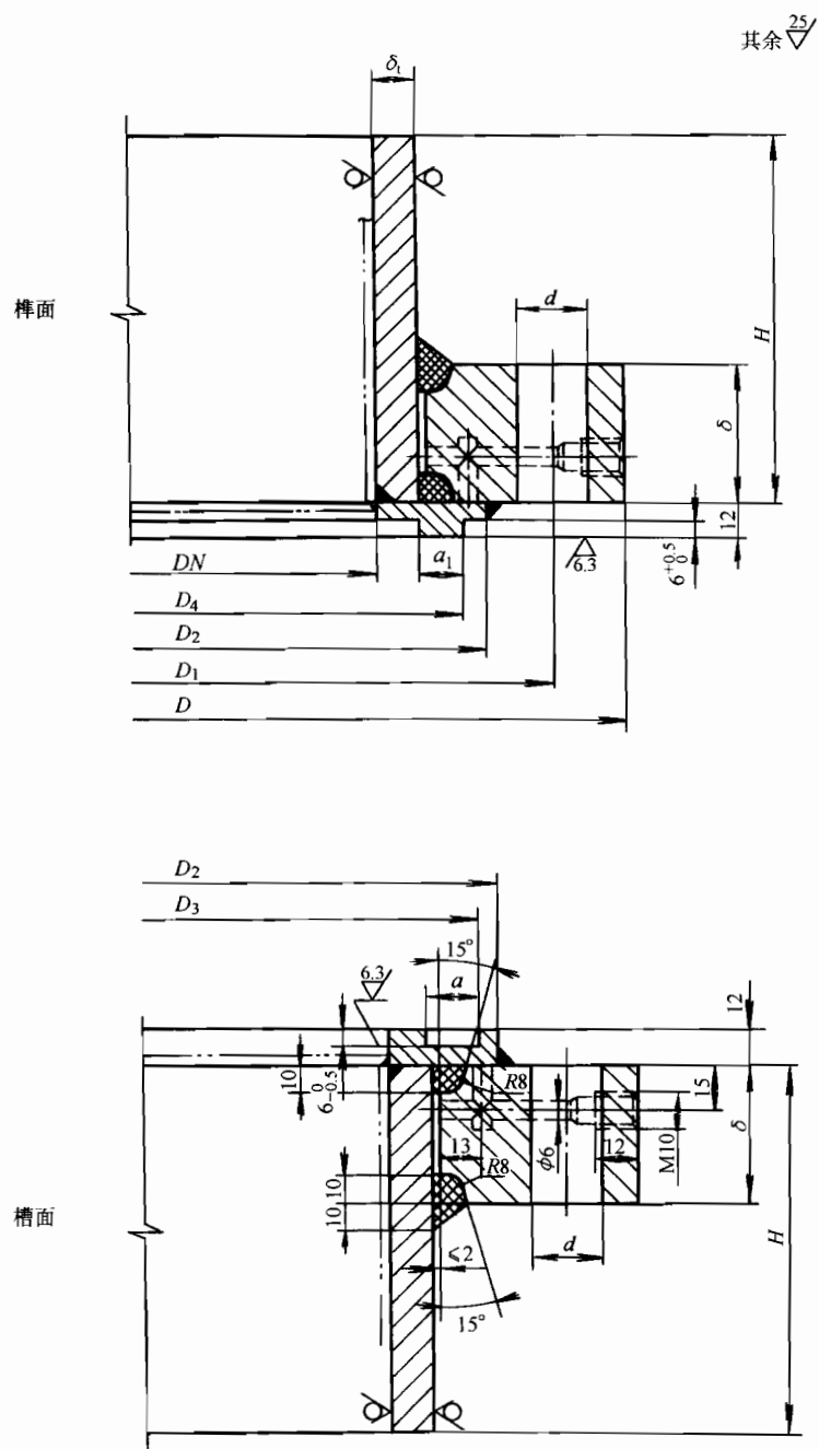
图 6 衬环棒槽密封面
